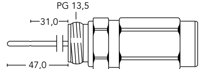
PG13,5m-XX
